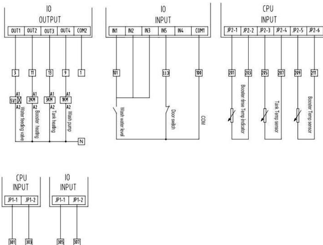
Diagrama do painel de controle
